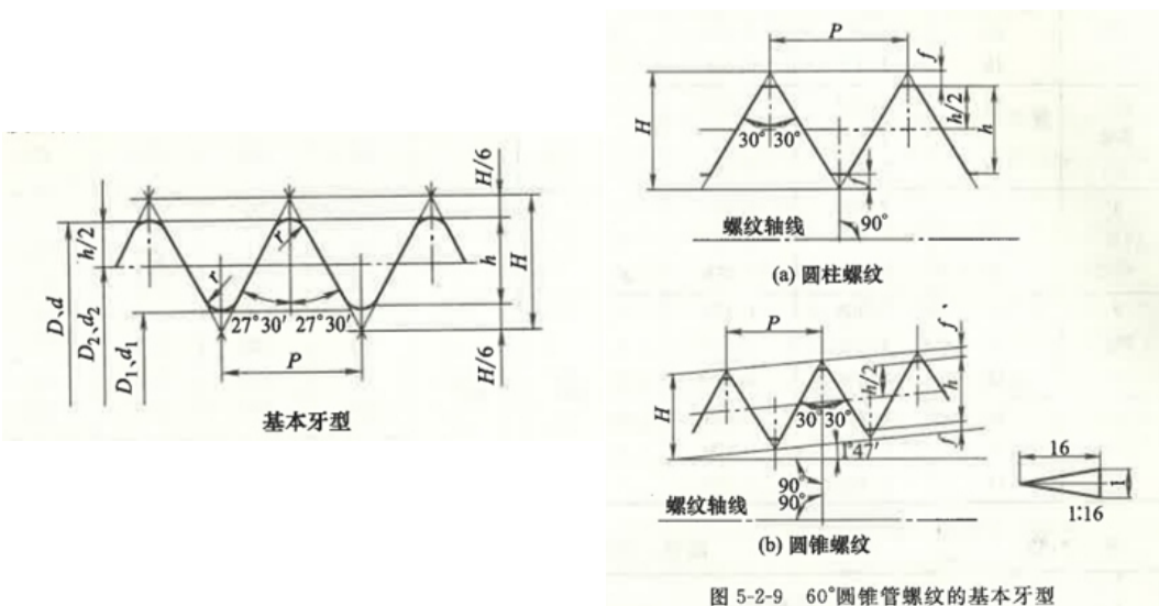
图 5-2-9 60°圆锥管螺纹的基本牙型
